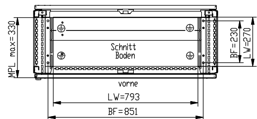
dreiteilige Bodenplatte frei einteilbar
