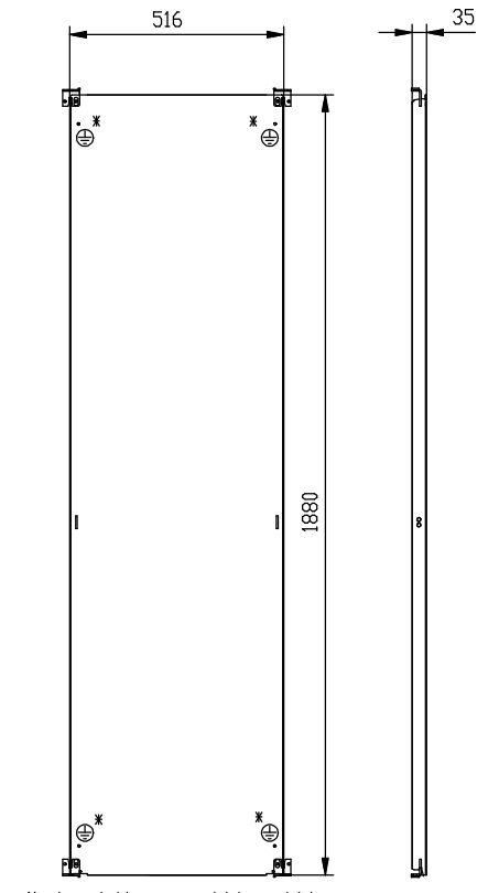
Montageplatte sendzimirverzinkt Blechstärke: 2,5 mm
