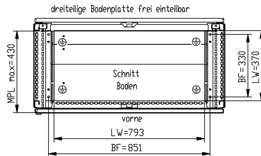
dreiteilige Bodenplatte frei einteilbar
