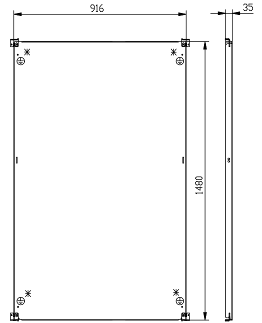
Montageplatte sendzimirverzinkt Blechstärke: 3,0 mm
