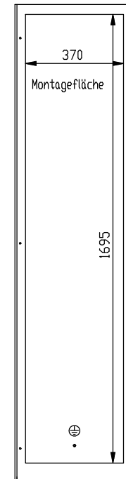
Seitenwand
